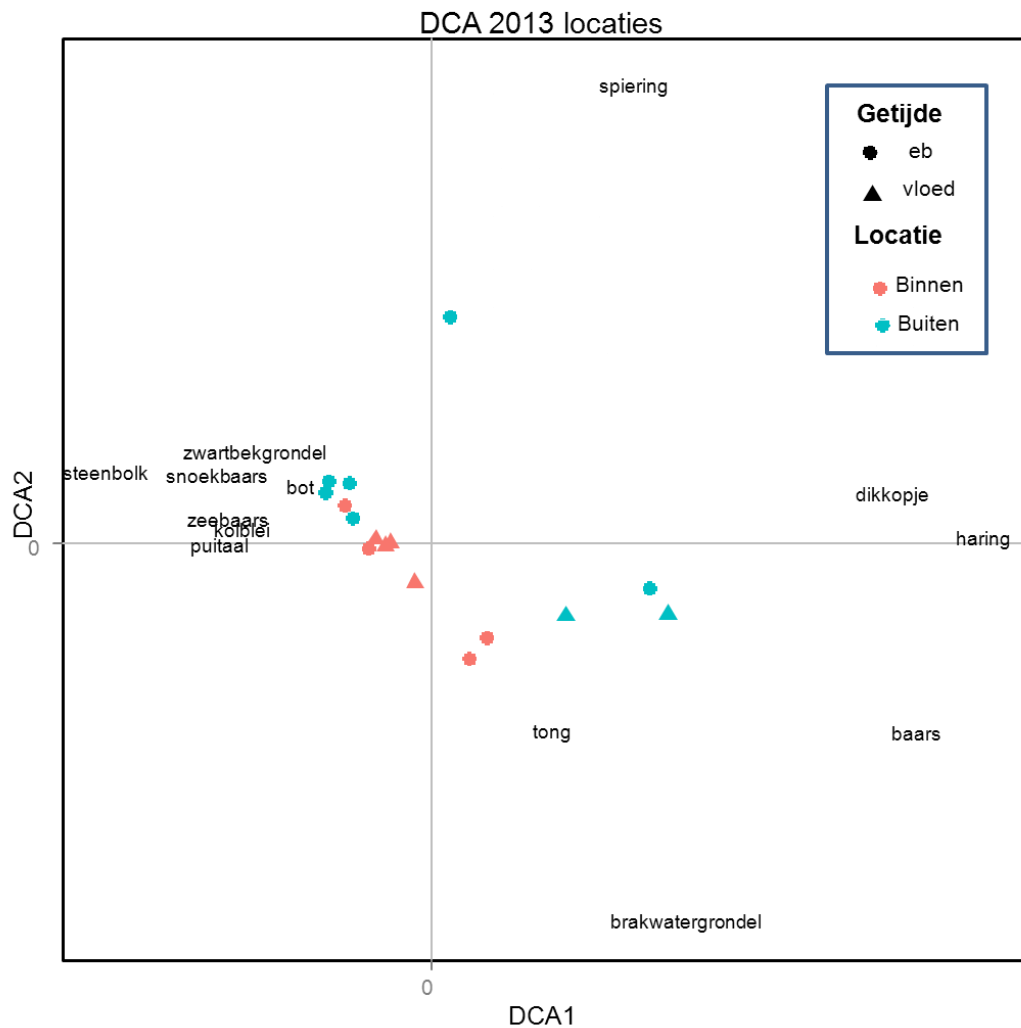
Figuur 10 NMDS ordinatie met relatieve abundantie gegevens (n= 16) van boomkorvangsten binnen en buiten de strekdams tijdens eb en vloed (eigenwaarden eerste en tweede as 0.3 en 0.18)
