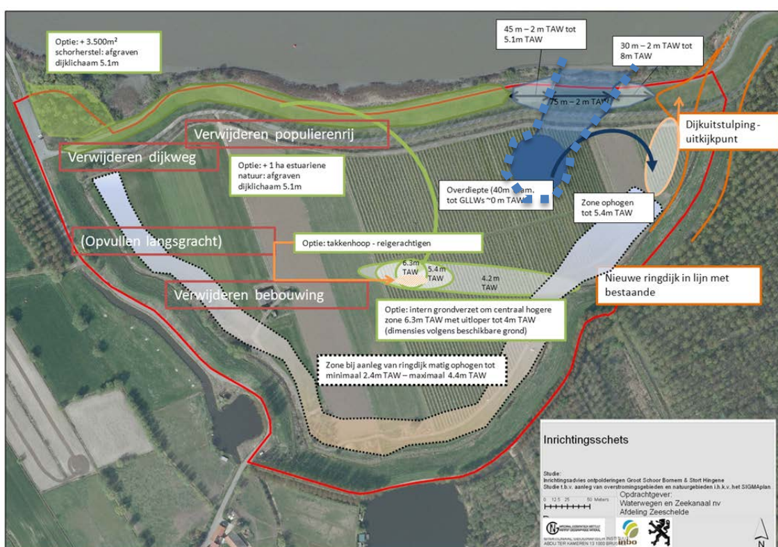
Figuur 1: Inrichtingsvoorstel Groot Schoor Bornem (Van Ryckegem et al., 2014). De blauwe geblokte contour toont de zone waar een beperkte kreekinsnijding verwacht wordt in de bodem.
